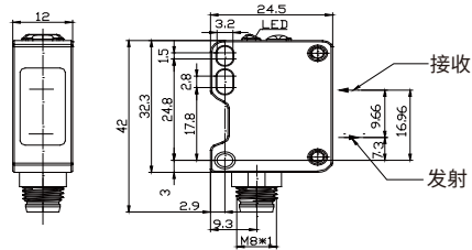
M8 连接器
