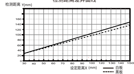
检测距离差异曲线
