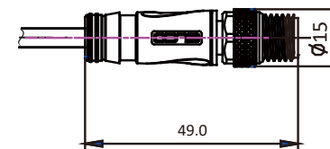
M12连接器
