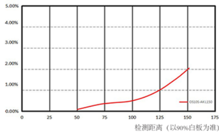
检测距离差异曲线(白90%黑6%)
