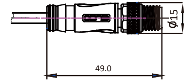
M12连接器
