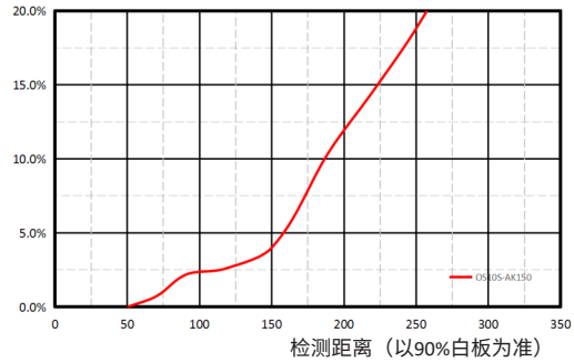
检测距离差异曲线 (白90%黑6%)
