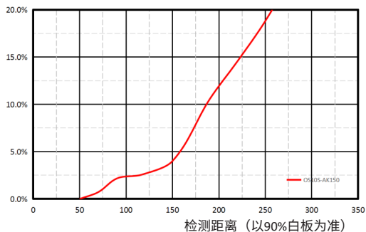
检测距离差异曲线 (白90%黑6%)
