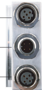
总线接口 2 LINK2-Bus out
