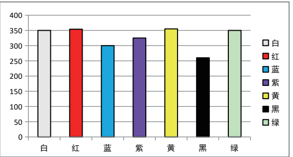
OS10S-AK350 颜色衰减图
