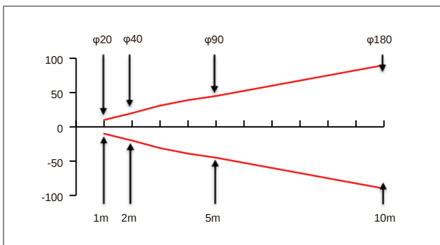
OS10S-AK350 光斑图 (mm)
