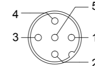
信号口 孔端
