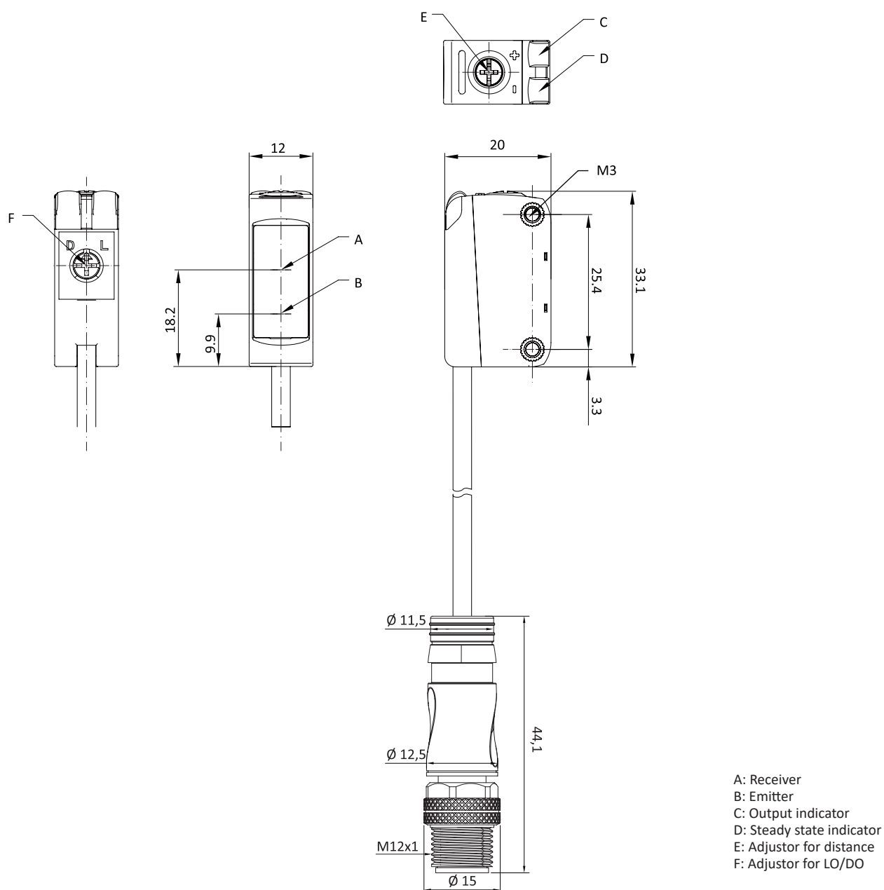
Fig. 3 BGS
