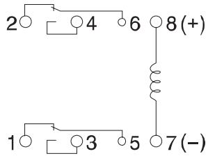
Fig. 1. WIRING DIAGRAM
