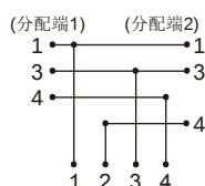
标准品电路图
